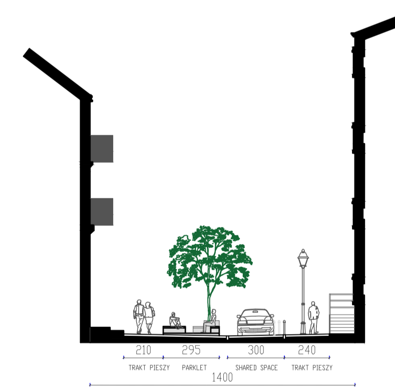
Przekrój A-A w skali 1:200
